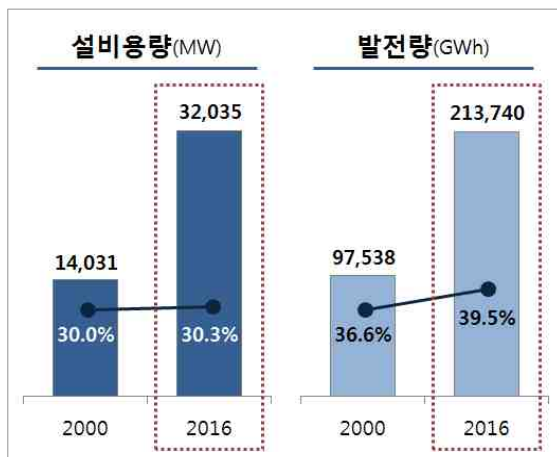
< 석탄화력발전 설비용량 및 발전량 추이 >
