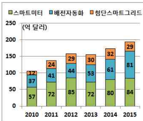
< 세계 스마트그리드 투자 규모 >
